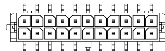
2*11PIN
