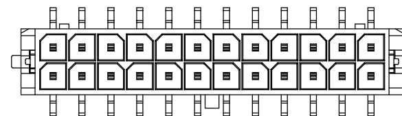
2*12PIN
