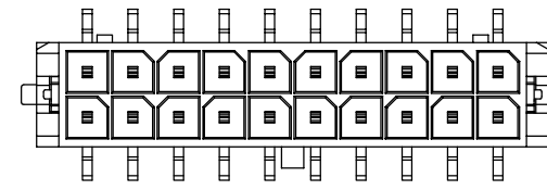
2*10PIN
