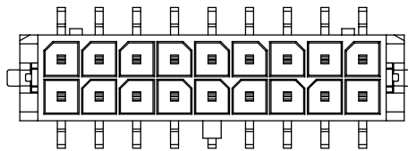
2*09PIN
