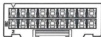
2*09P
