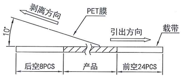
(PET膜剥离示意图)
