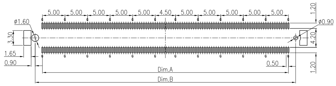
Reference P.C.B Layout
